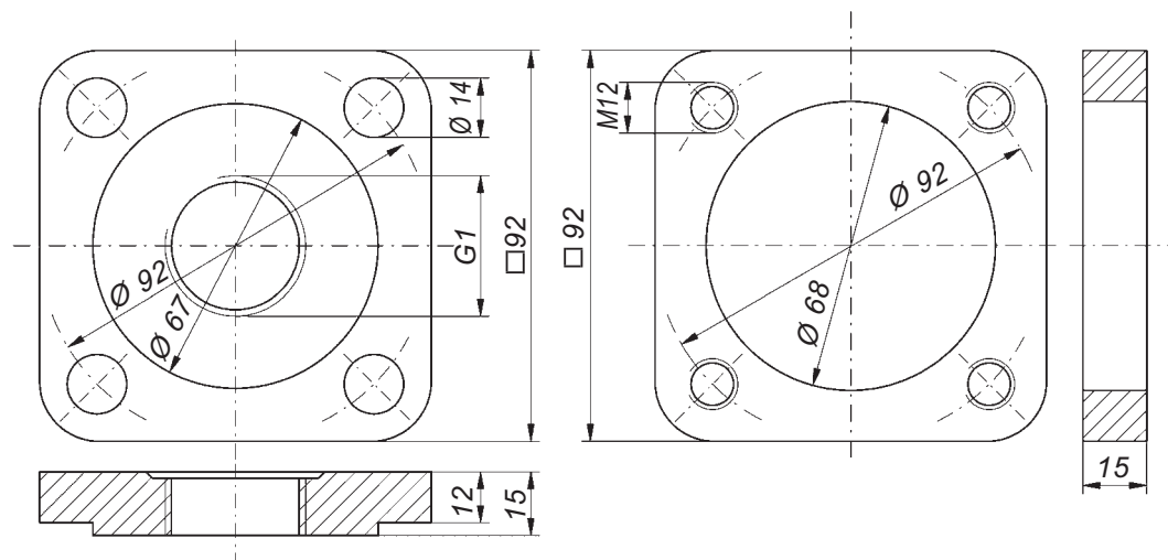
Vierkantflansch
